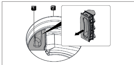
Abb. 9.4 Filterwechselklappe entfernen
