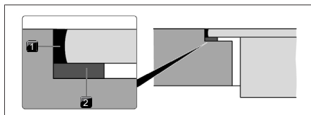
Abb. 11.18 Dichtungsband bei flächenbündiger Montage
