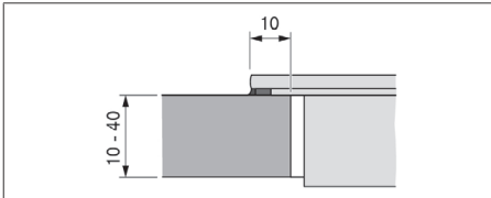
Abb. 11.8 Auflagemaß für Aufsatzmontage
