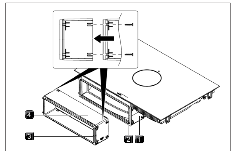
Abb. 11.15 Verlängerung des Teleskopauszuges
