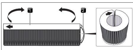
Abb. 9.7 Geruchsfilter
