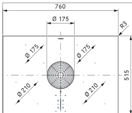
Abb. 3.4 PURU2/R Gerätemaße Draufsicht
