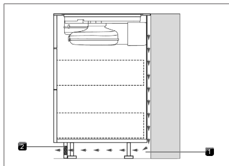
Abb. 11.10 Rückströmöffnung im Sockelbereich
