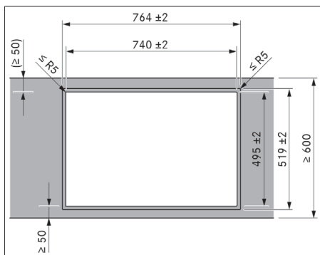
Abb. 11.5 Ausschnittsmaße für flächenbündige Montage
