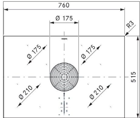
Abb. 3.1 PURA2/R Gerätemaße Draufsicht
