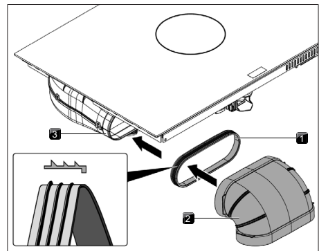
Abb. 11.24 Anschluss an Kanalsystem
