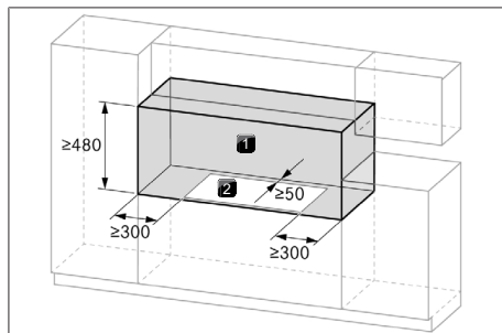
Abb. 11.3 Erforderlicher Freiraum
