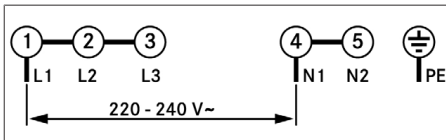
Abb. 11.28 Anschlusschema 1-Phasen-Anschluss
