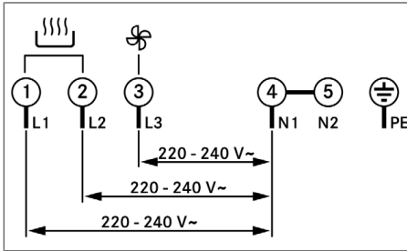
Abb. 11.27 Anschlusschema 3-Phasen-Anschluss
