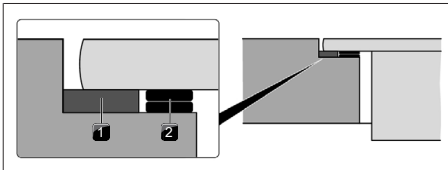
Abb. 11.22 Höhenausgleichsplatten
