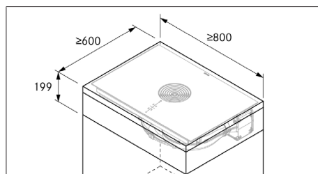
Abb. 11.4 Möbel-Mindestmaße
