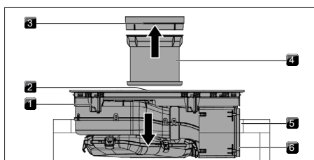
Abb. 11.20 Kochfeld mittig einsetzen
