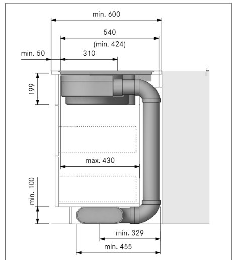
Abb. 11.9 Einbaumaße Abluft, Arbeitsplattentiefe 600 mm
