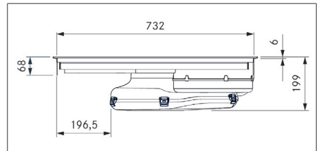
Abb. 3.2 PURA2/R Gerätemaße Vorderansicht
