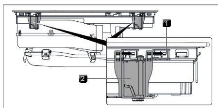
Abb. 11.19 Montageklappen anbringen
