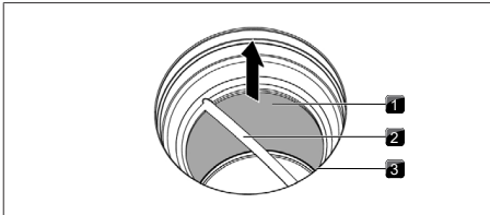
Abb. 9.2 Edelstahl-Fettfilter ausbauen
