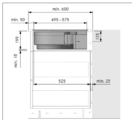
Abb. 11.16 Einbaumaße bei Umluft-Montagevariante B, Arbeitsplattentiefe 600 mm
