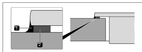
Abb. 11.17 Dichtungsband bei Aufsatzmontage
