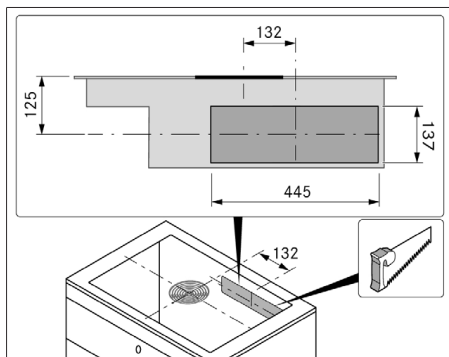
Abb. 11.11 Rückwand-Ausschnitt
