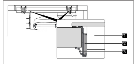
Abb. 11.23 Kochfeld mittig befestigen
