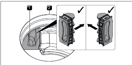
Abb. 9.10 Filterwechselklappe einsetzen
