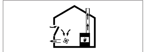
Abb. 11.2 Abluftmontage – korrekt
