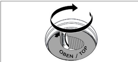
Abb. 9.9 Geruchsfilter in Endposition platzieren
