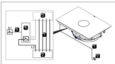
Abb. 11.26 Anschlussschema mit externem Schaltkontakt
